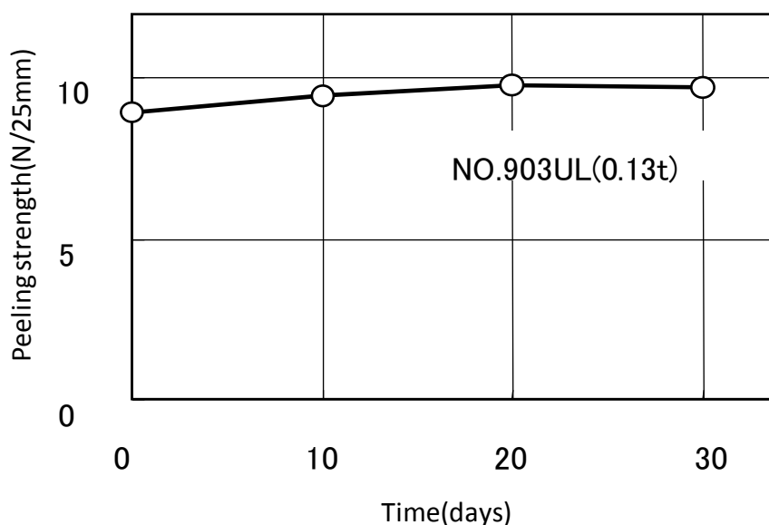
図 2 引き剥がし粘着力の耐熱性（180℃）
